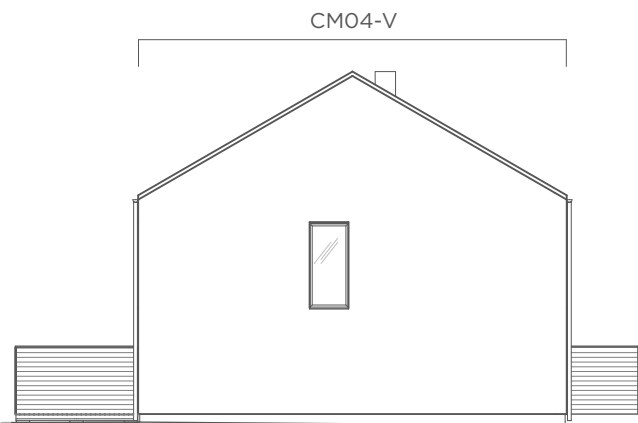
VÄNSTER GAVEL
