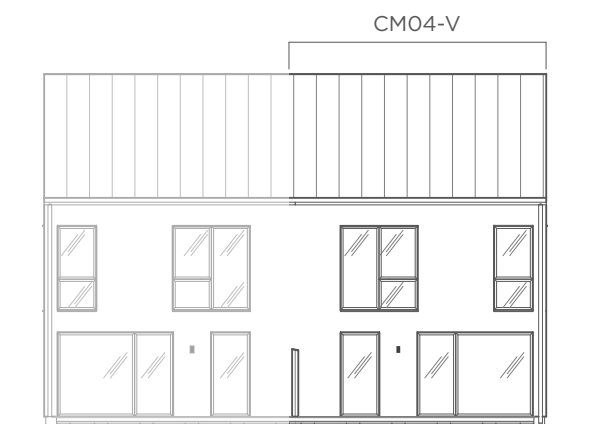
FASAD MOT TRÄDGÅRD
