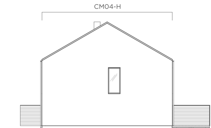
HÖGER GAVEL
