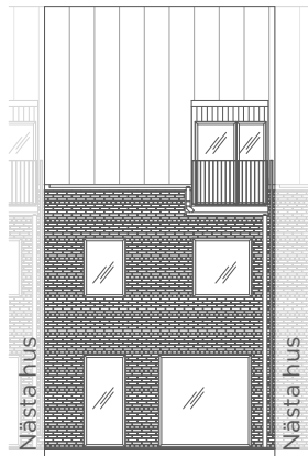
FASAD TRÄDGÅRDSSIDA
