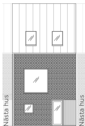
FASAD MOT GATA
