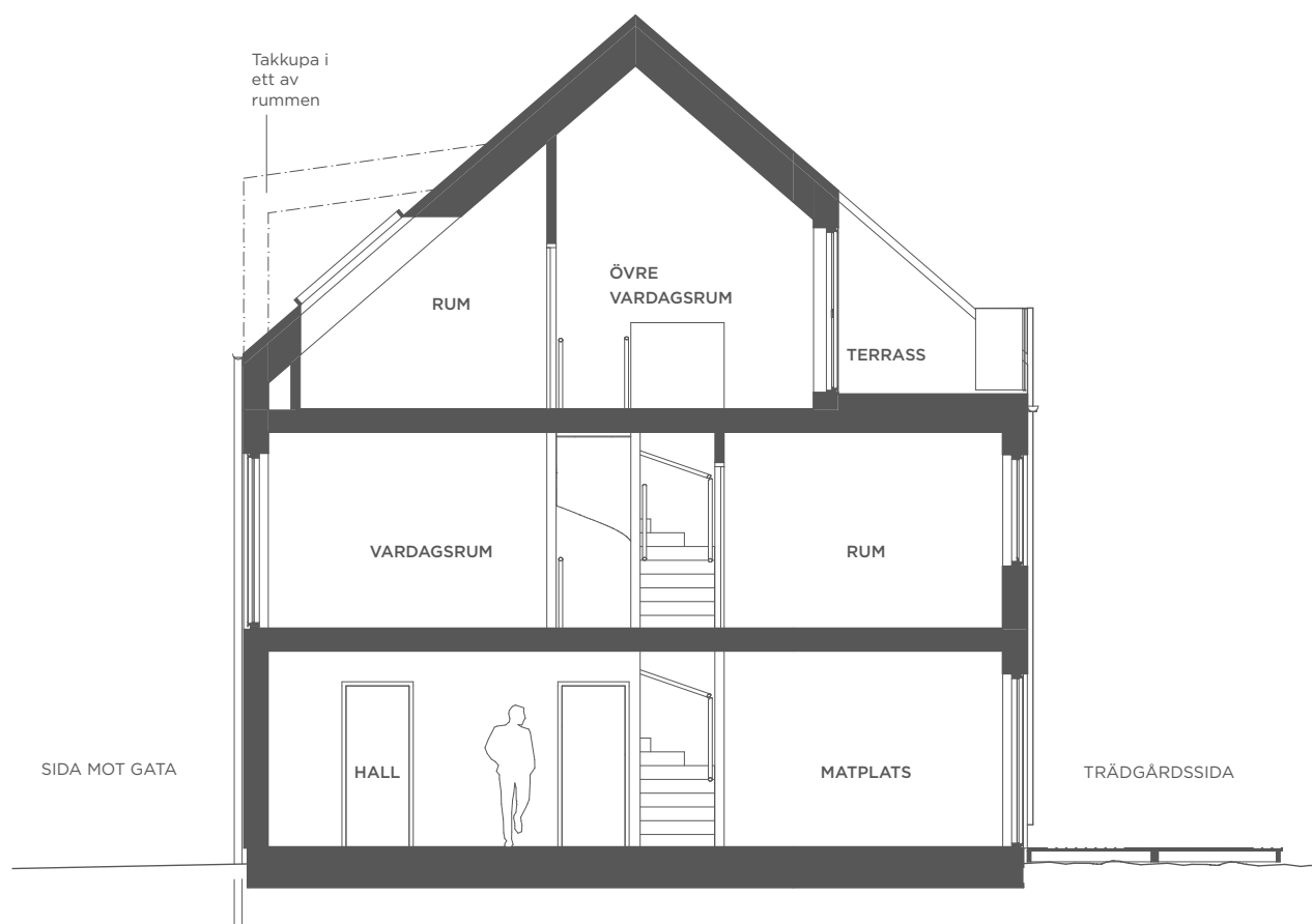
SEKTION
