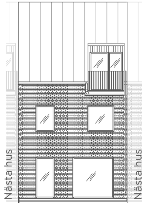
FASAD TRÄDGÅRDSSIDA
