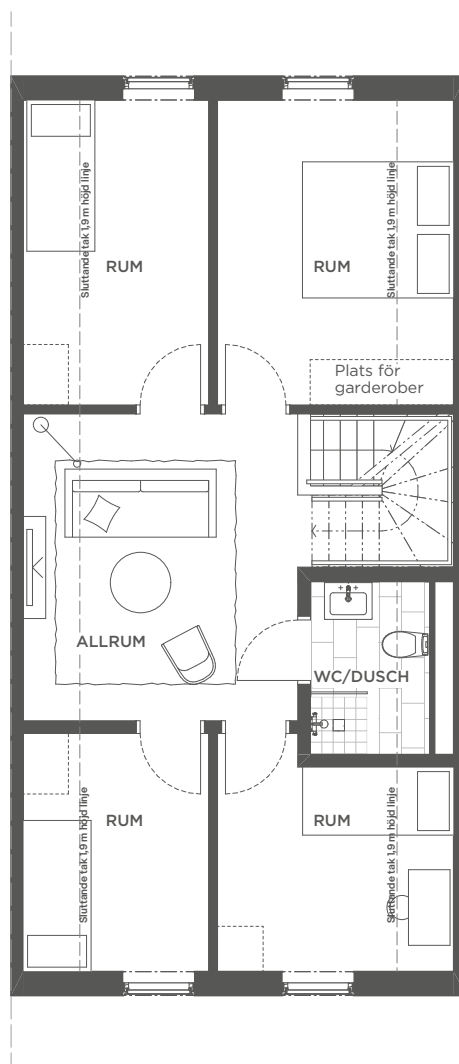
ÖVRE PLAN
