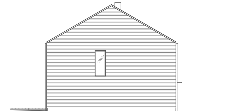
VÄNSTER GAVEL
