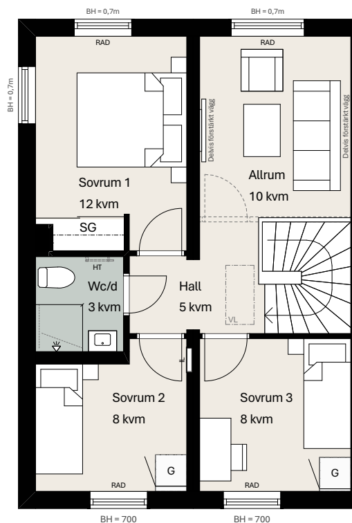
Plan 2 - Överplan
