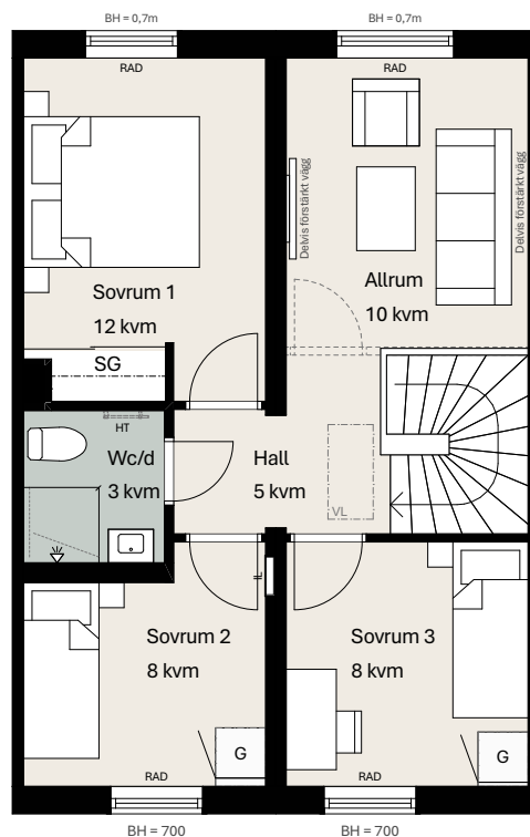
Plan 2 - Överplan
