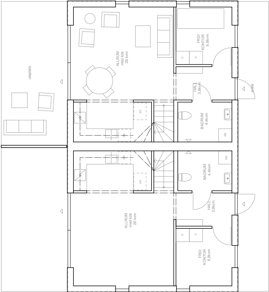
ENTRÉPLAN 44 kvm (44,3) villalägenhet
