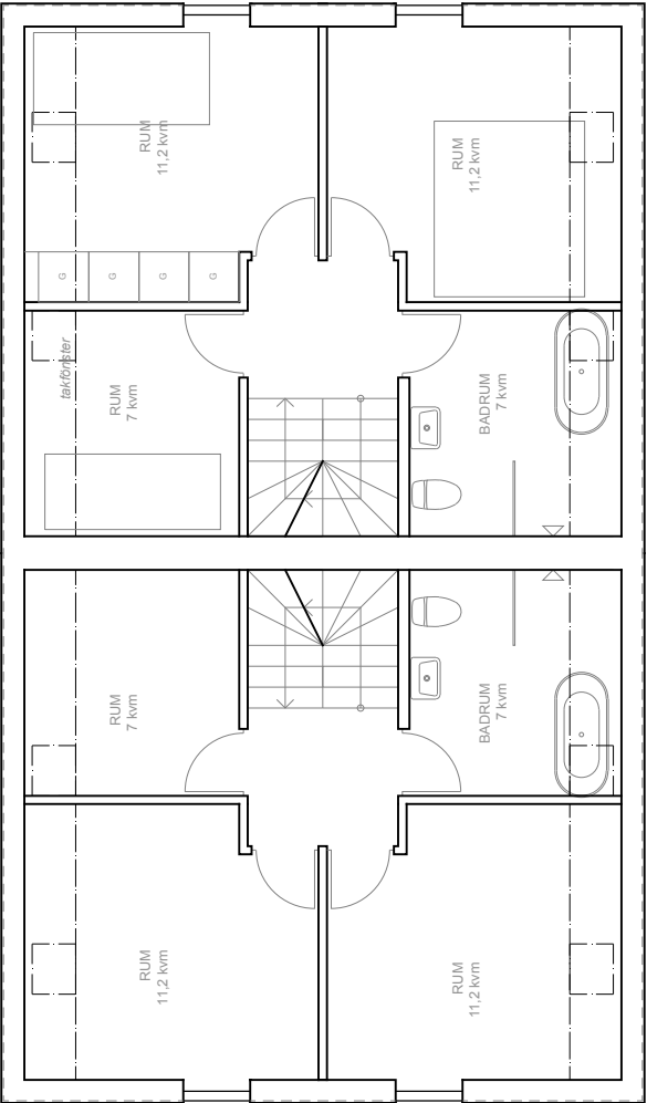
MELLANPLAN 44kvm (43,7) villalägenhet
