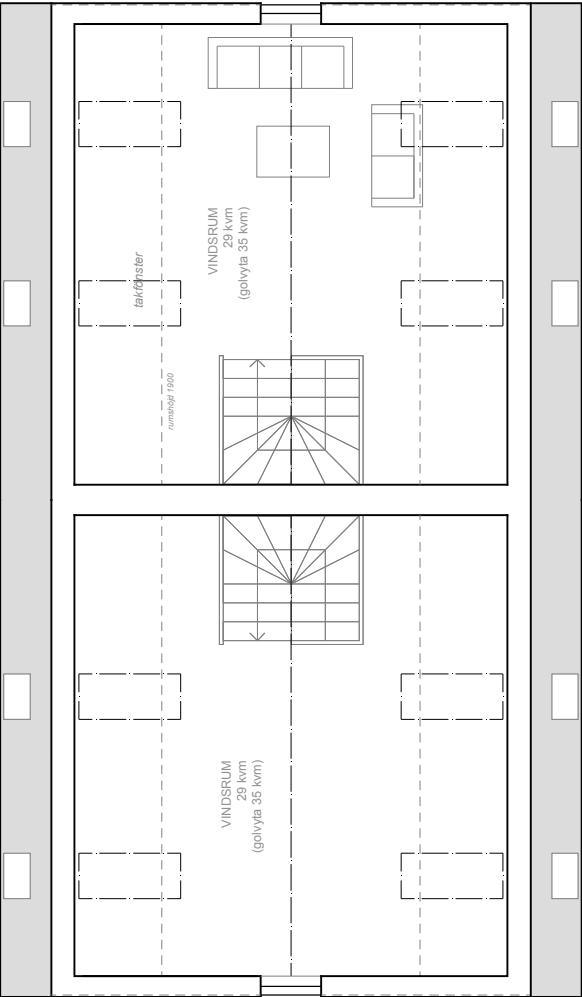
VINDSPLAN 29 kvm (28,6/35) villalägenhet
