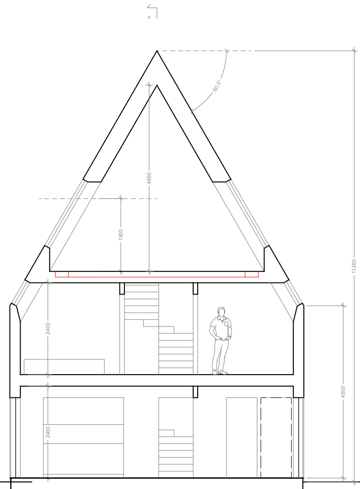
SEKTION C-C
