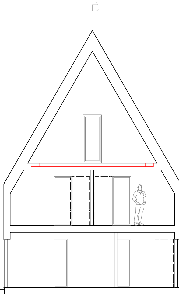
SEKTION B-B
