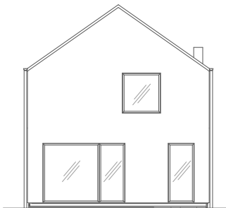
FASAD TRÄDGÅRDSSIDA
