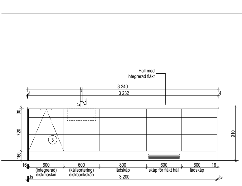
C-C ELEVATION KÖKSÖ MOT KÖK
