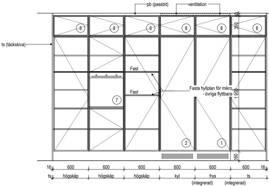
A-A ELEVATION
