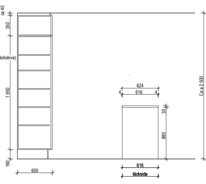
B-B ELEVATION-SEKTION
