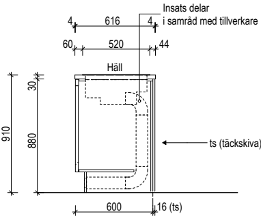
E-E SEKTION GENOM KÖKSÖ
