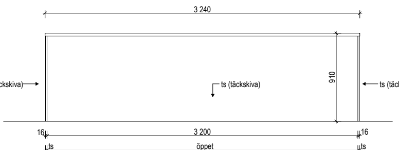
D-D ELEVATION KÖKSÖ
