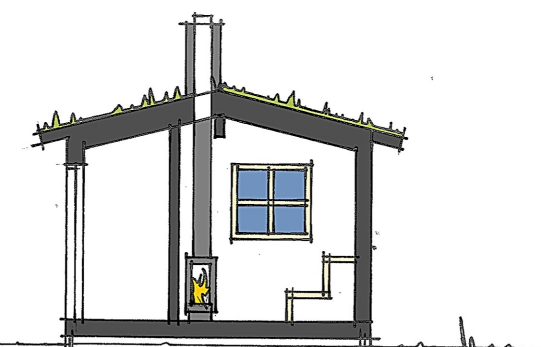
SEKTION
