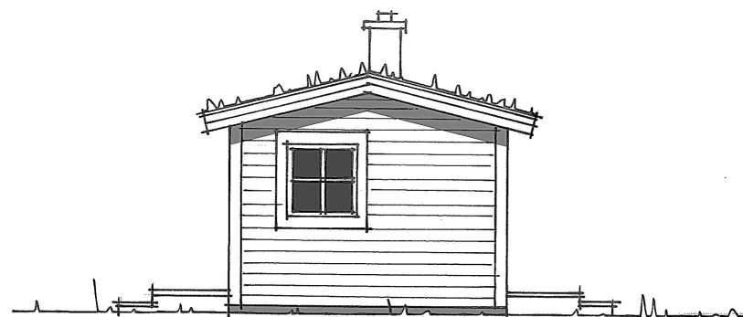
FASAD MOT SÖDER - HAVET
