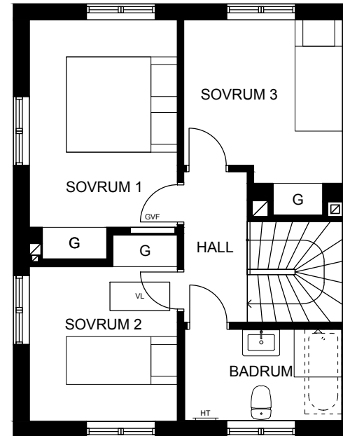
ÖVRE PLAN
