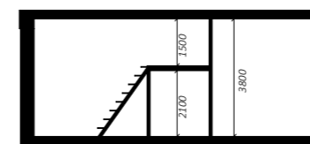
SEKTION SKALA 1:200 ALLA MÅTT ÄR CIRKA MÅTT
