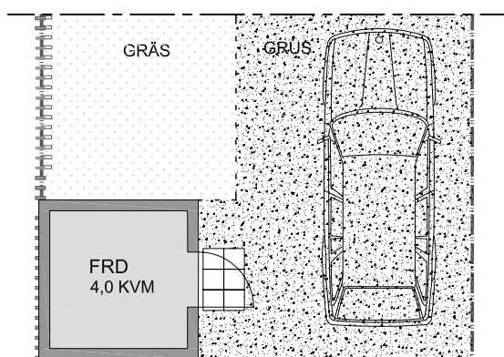
Bottenvåning 56,4kvm
